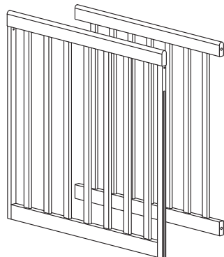
Решетка передняя, 1 шт. Решетка задняя, 1 шт.
